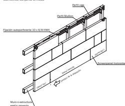
Instalación Screenpanel J Isométrica conjunto armado
